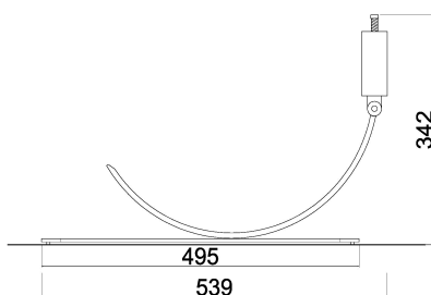
ALZADO
