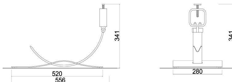
ALZADO
