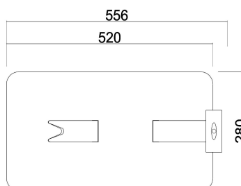
JAMONERO. PLANTA.
