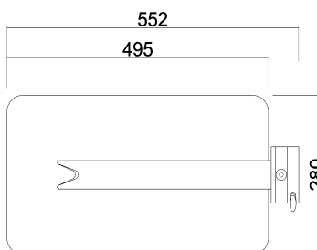
JAMONERO. PLANTA.
