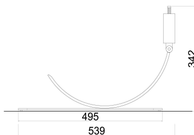
ALZADO
