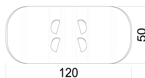
PIEZA EN "V". VISTA INFERIOR
