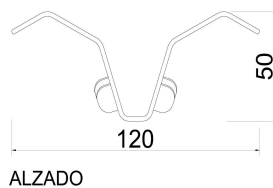
ALZADO
