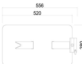
JAMONERO. PLANTA.
