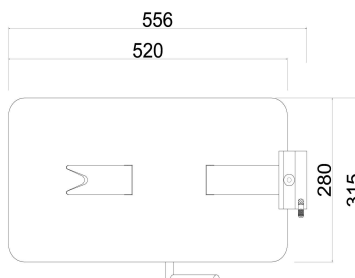
JAMONERO. PLANTA.
